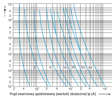
Pasmo czasowo-prądowe wkładek topikowych typu „gG”
