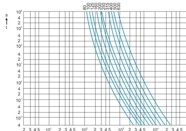
Prąd zwarciaowy spodziewany (wartość skuteczna) Ip (A) (Prospective current (effective value), Ip (A))
