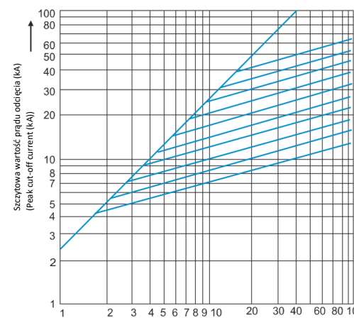
Prąd zwarciaowy spodziewany Ip (kA), wartość skuteczna – symetryczna (Prospective current Ip (kA) (symmetrical effective value))
