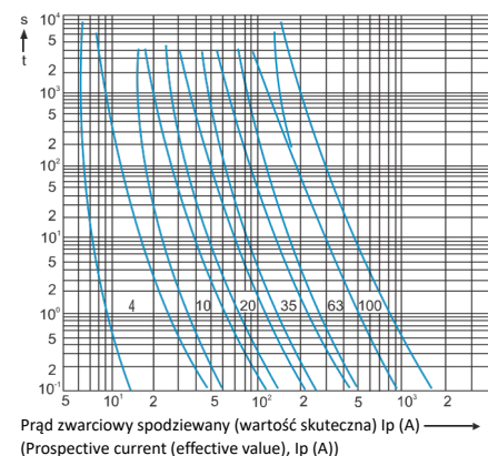
Pasmo czasowo-prądowe wkładek topikowych typu „gG”
