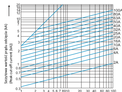
Prąd zwarciaowy spodziewany Ip (kA), wartość skuteczna – symetryczna (Prospective current Ip (kA) (symmetrical effective value))
