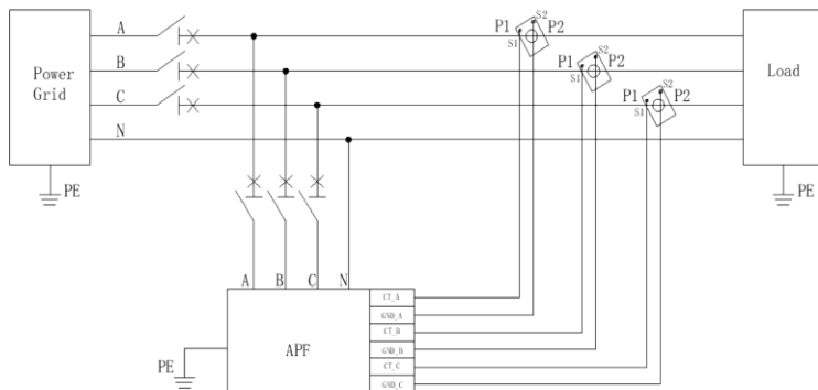
Schemat podłączenia
