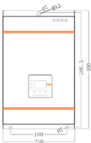
Wymiary ogólne
